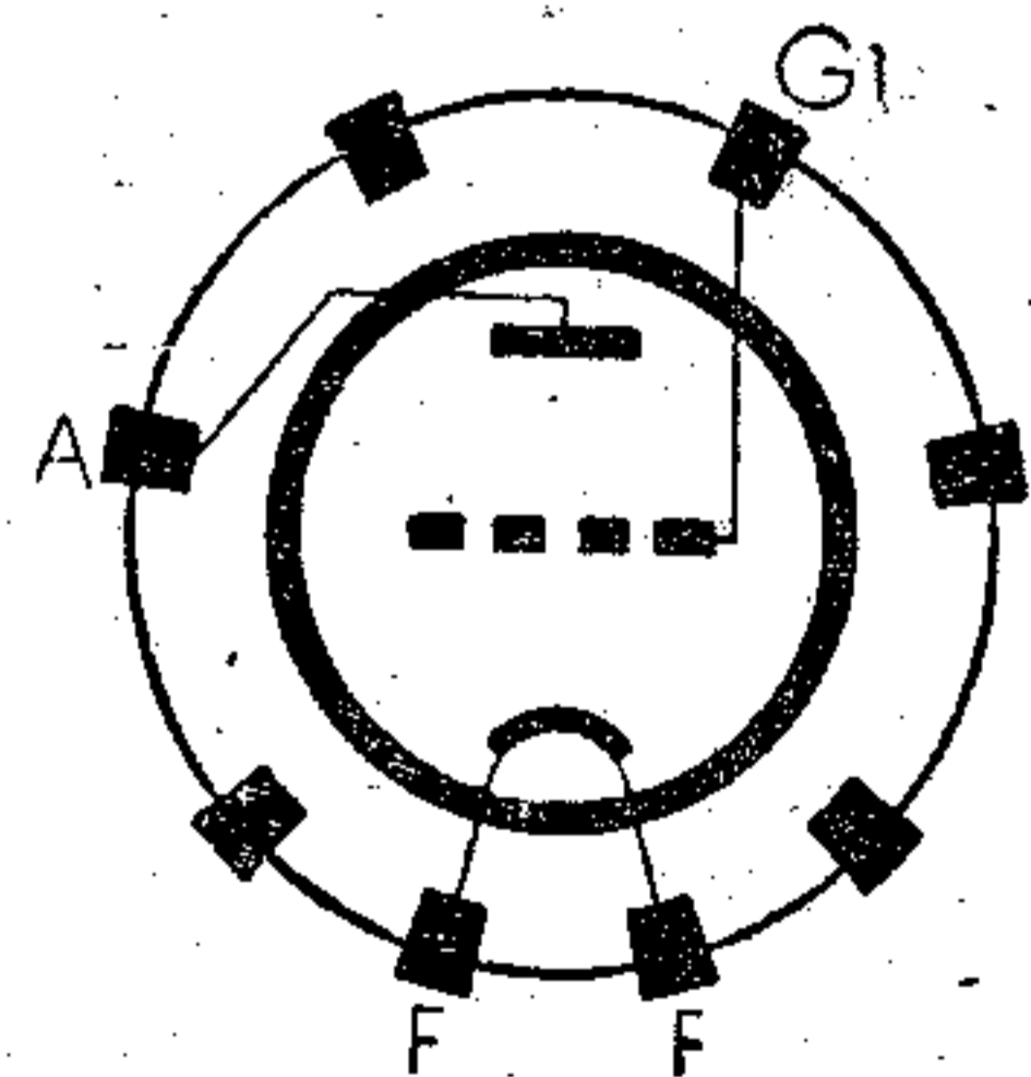
Sockelschaltung
